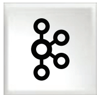
Apache Kafka
